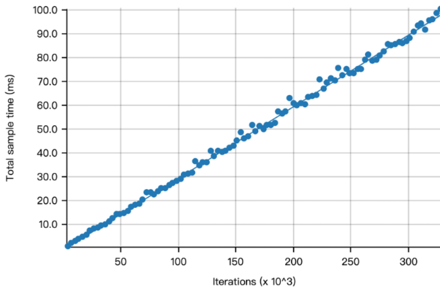
图 6 消息编码速率拟合曲线
