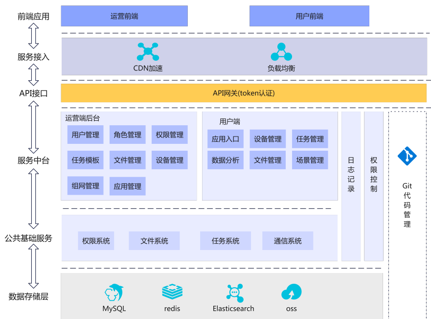
图 2 平台主体结构
