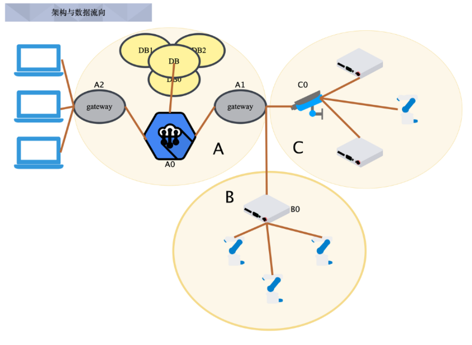
图 2 系统结构图
