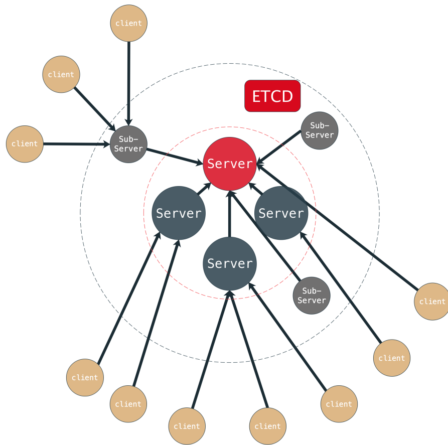
图 5 通讯网络
