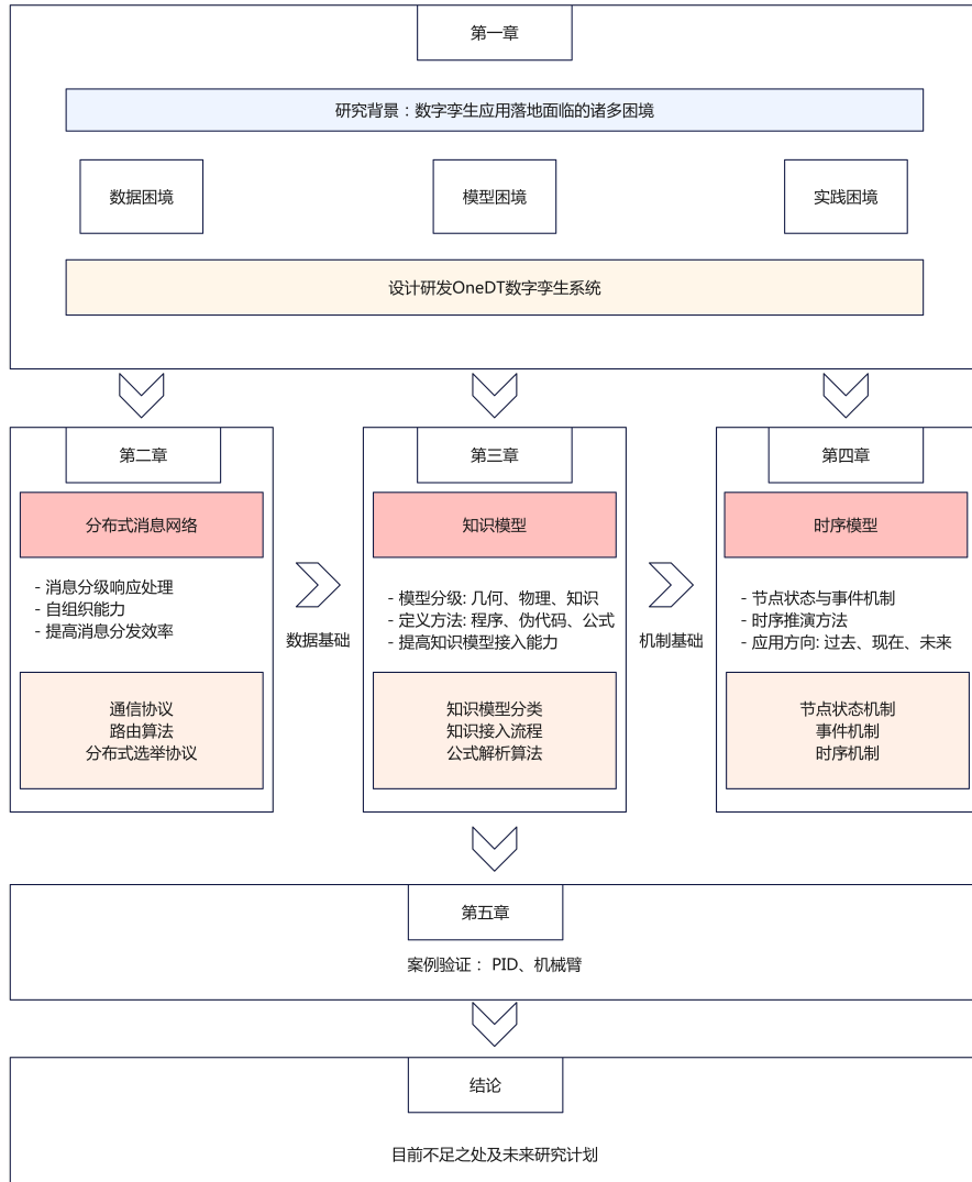
图 1 文章结构图
